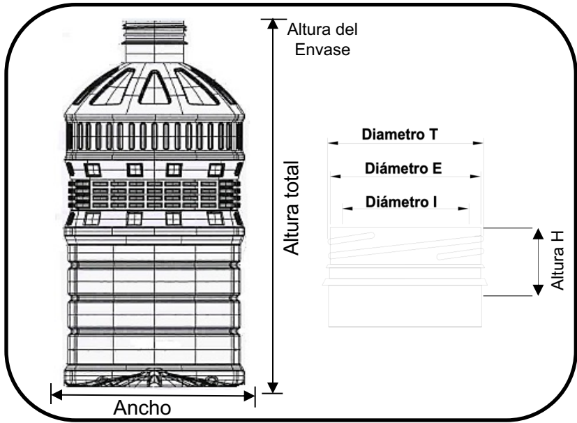
Plano Mecánico
