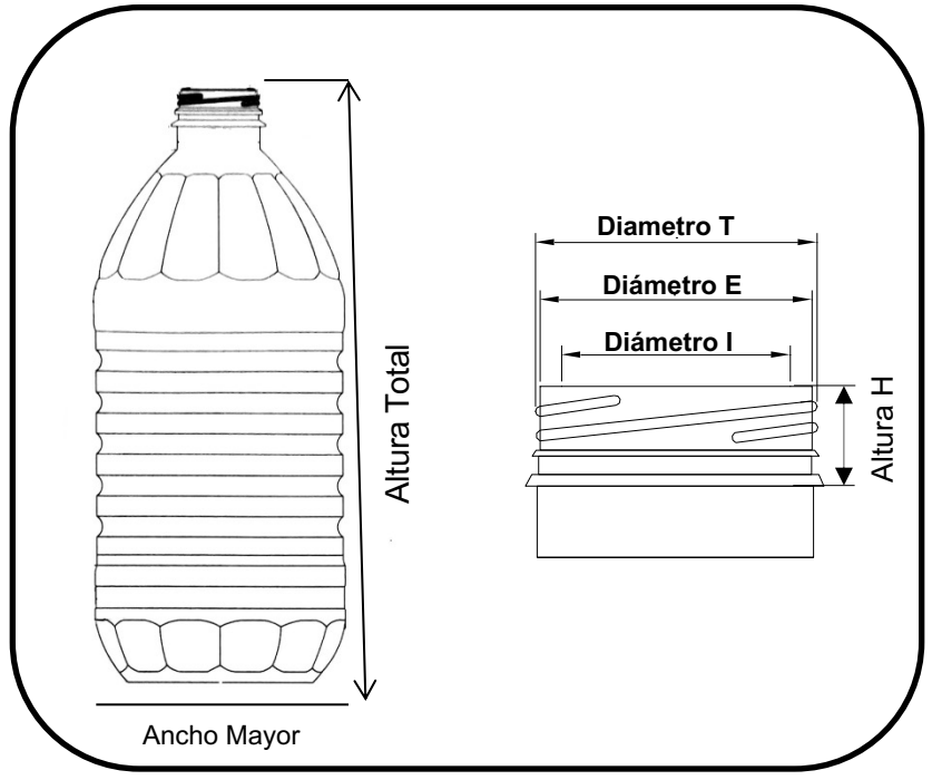
Plano Mecánico
