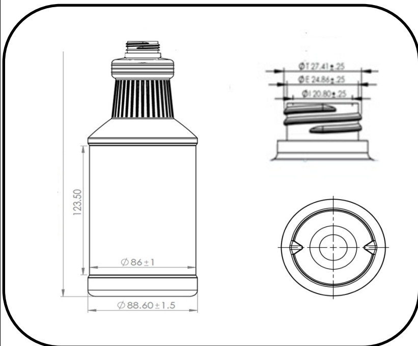
Plano Mecánico
