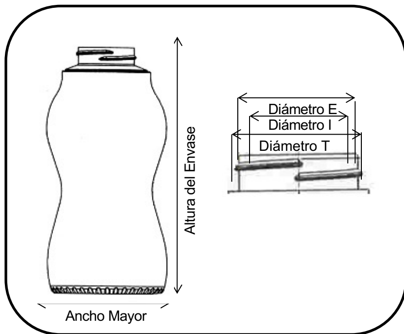
Plano Mecánico
